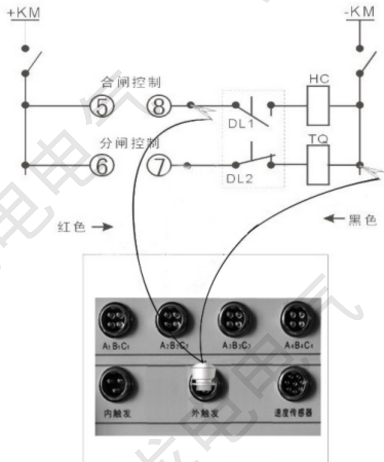
合闸外触发接线示意图
