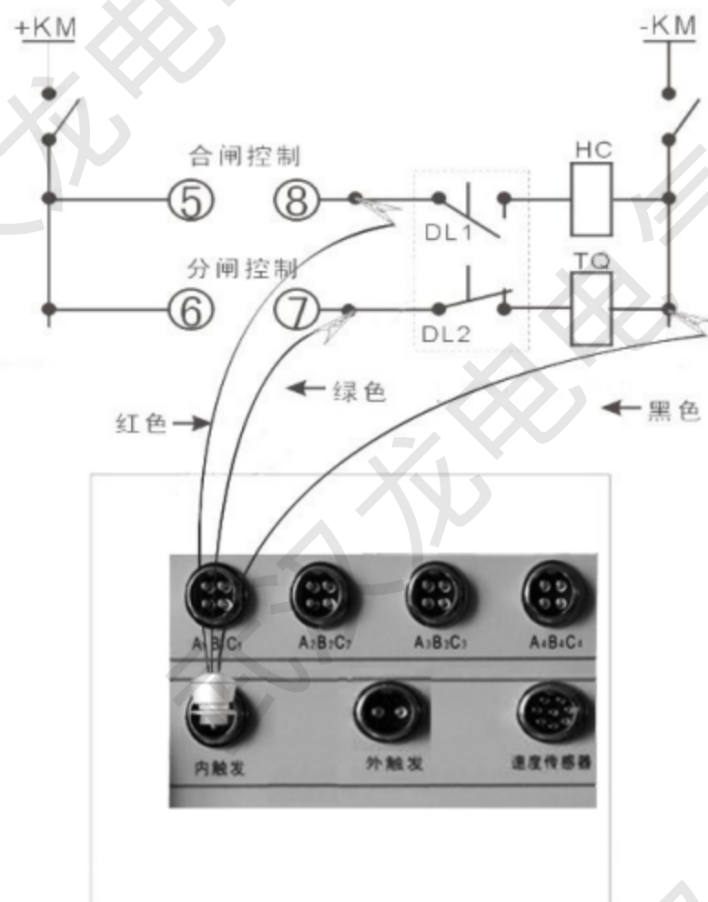
内触发控制接线示意图
