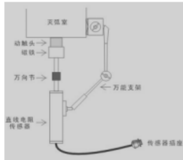
安装示意图
